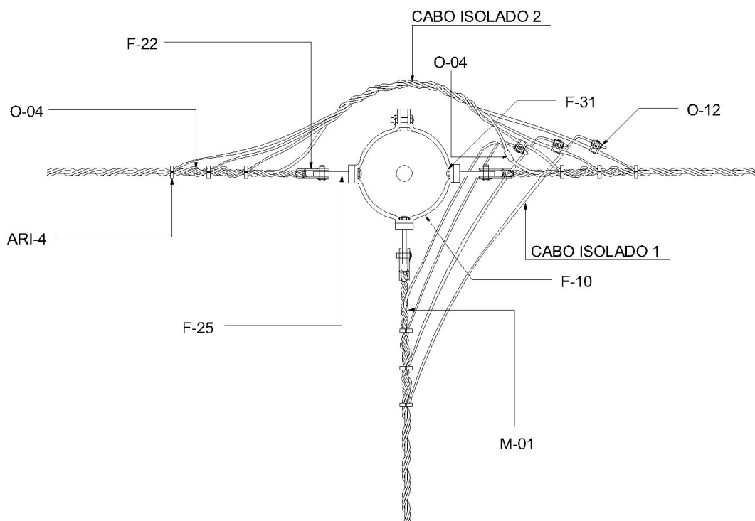
Figura 9 - Estrutura derivação SI 4 – SI 3
