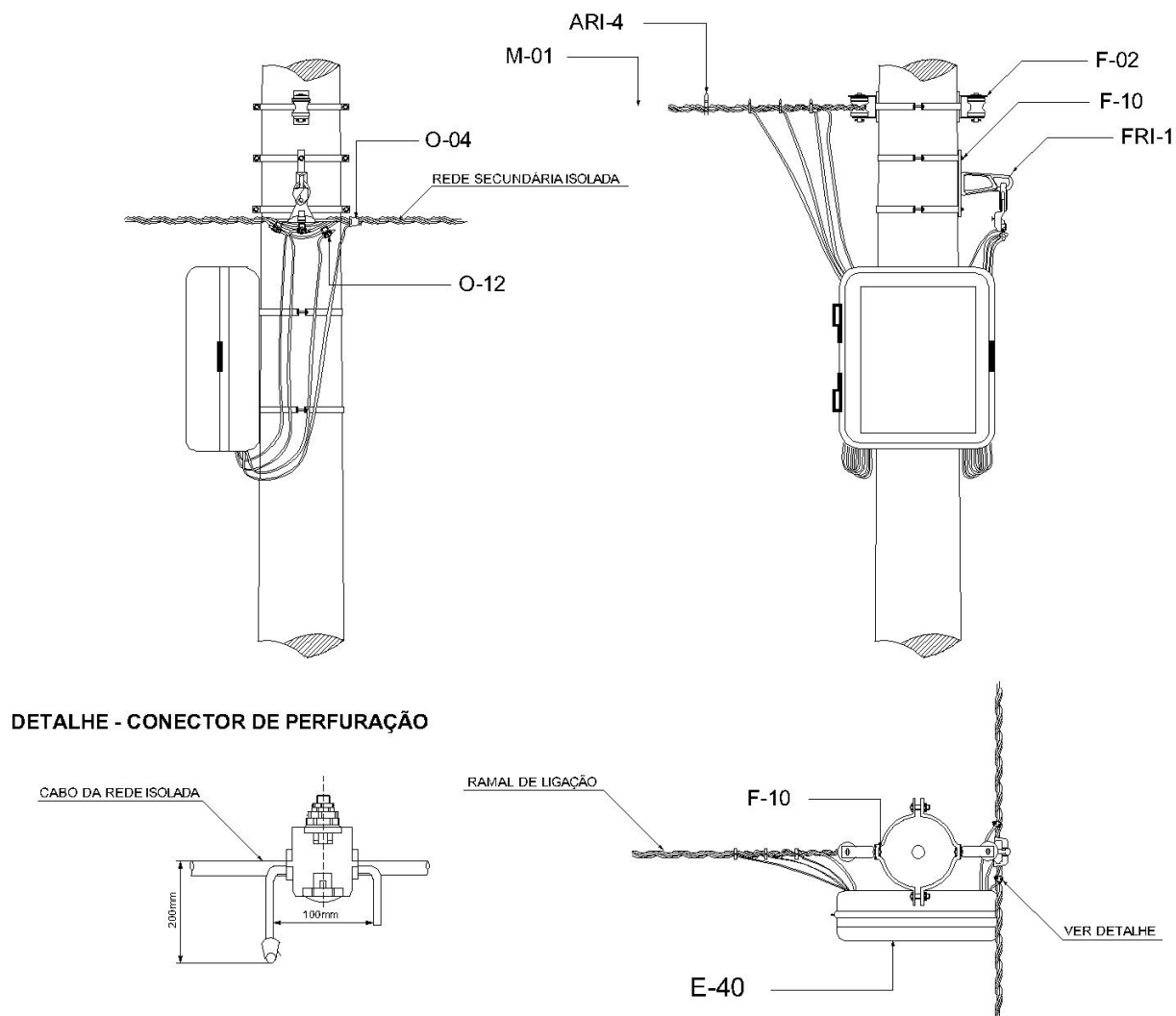
Figura 15 – Ramal de ligação - Caixa de ligações
