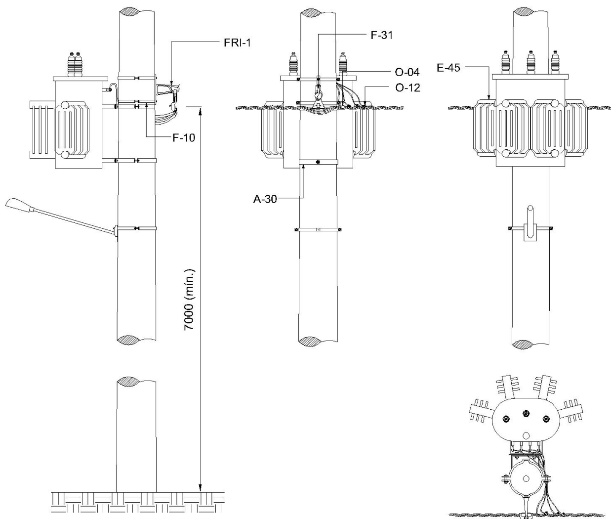
Figura 13 - Instalação de transformador SITR
