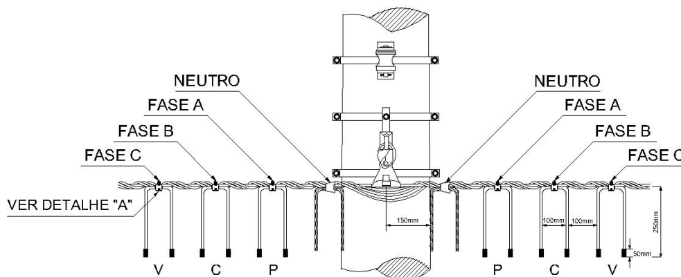
Figura 19 - Ramal de ligação –Várias conexões
