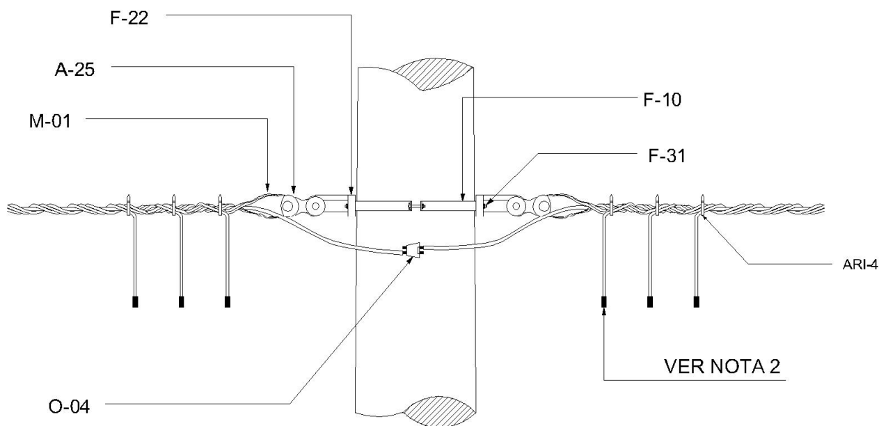
Figura 6 – Estrutura ancoragem sem Jumper SI 3 – SI 3
