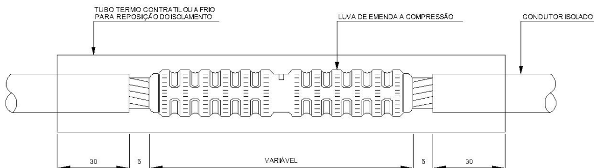
Figura 22 - Emenda reta do cabo - Maneira 1
