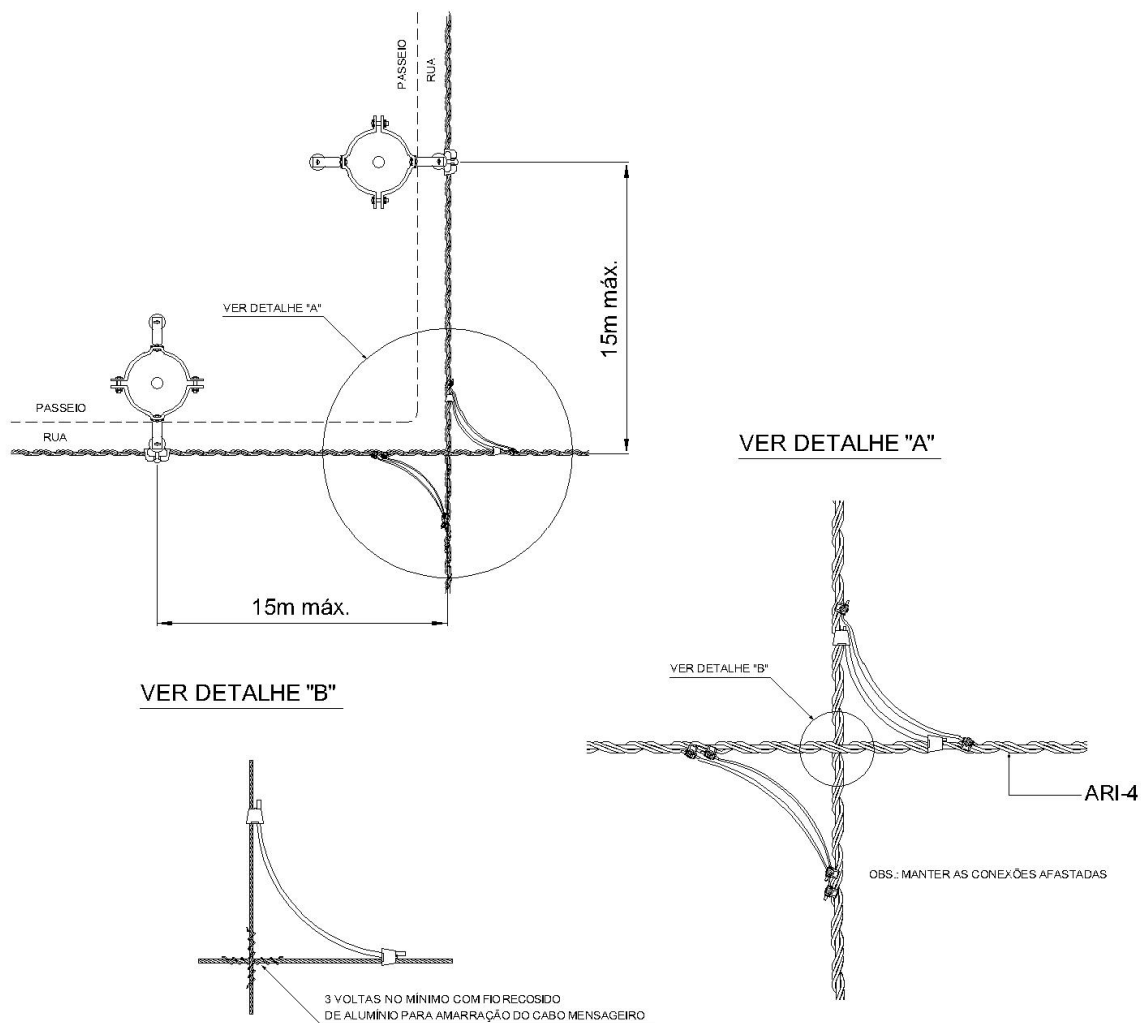
Figura 10 - Estrutura conexão no vão (FLYNG – TAP)
