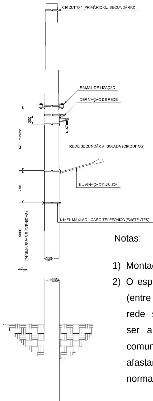
Figura 1 – Instalação básica
