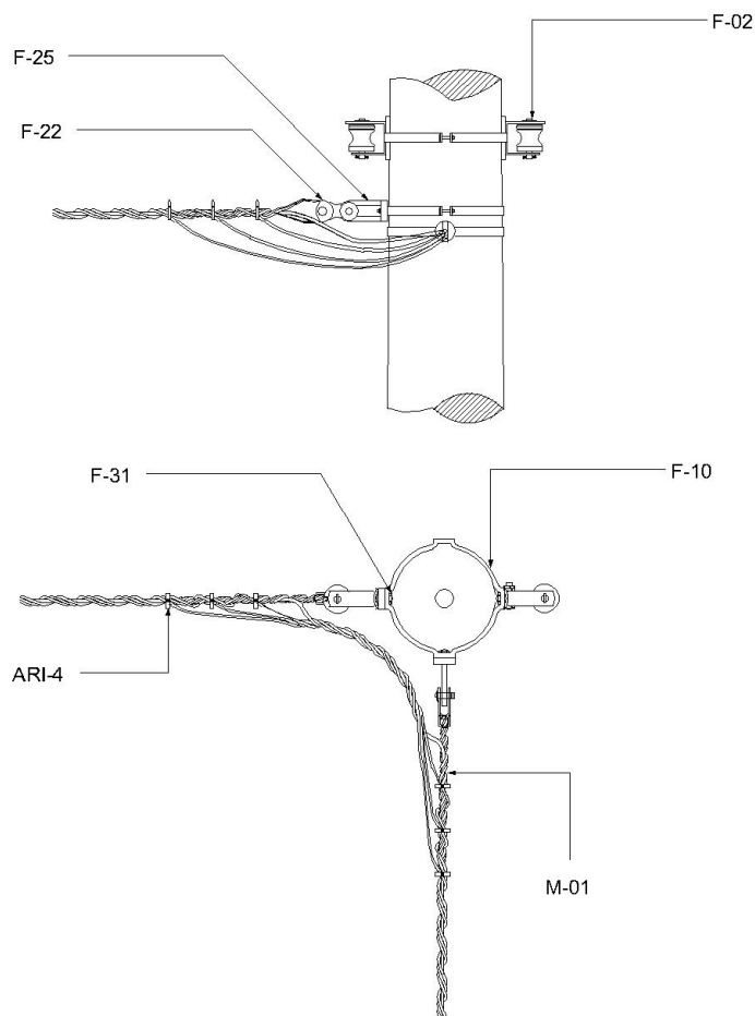
Figura 12 - Estrutura 90° - SI 11
