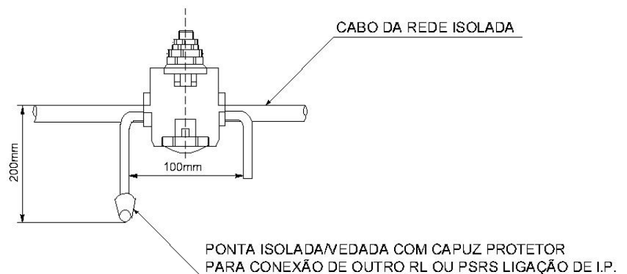
Figura 18 - Detalhe "B" - Conector de perfuração
