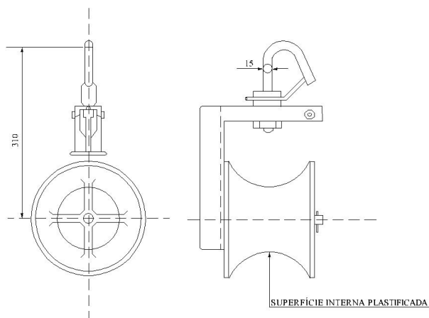
DESENHO 2 - ROLDANA
