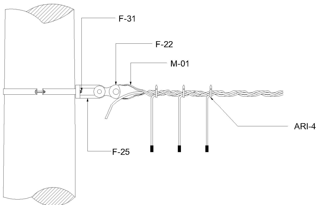
Figura 4 – Estrutura fim de rede – SI 3
