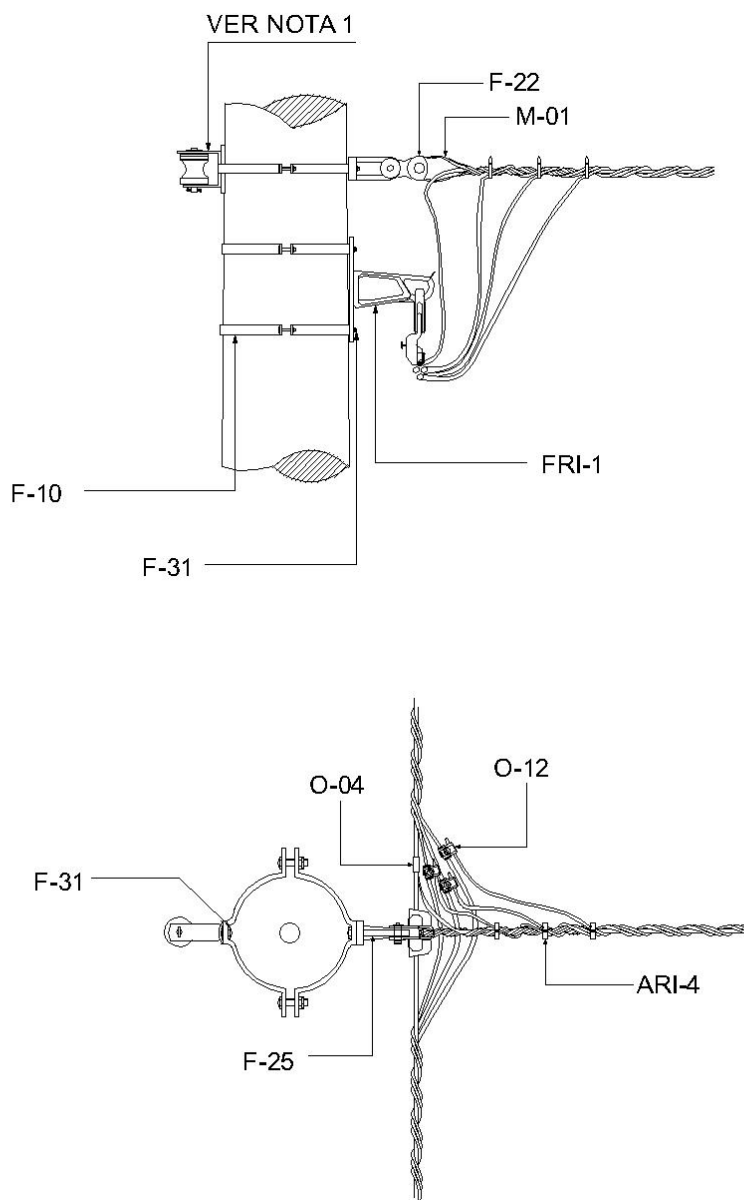
Figura 8 - Estruturas derivação tangente – SI 1 – SI 3
