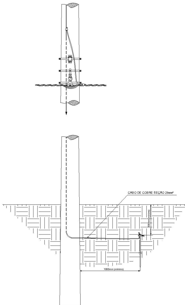
Figura 21 - Aterramento - Neutro
