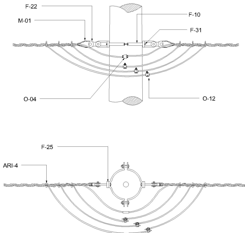
Figura 5 – Estrutura ancoragem com mudança de seção – SI 4
