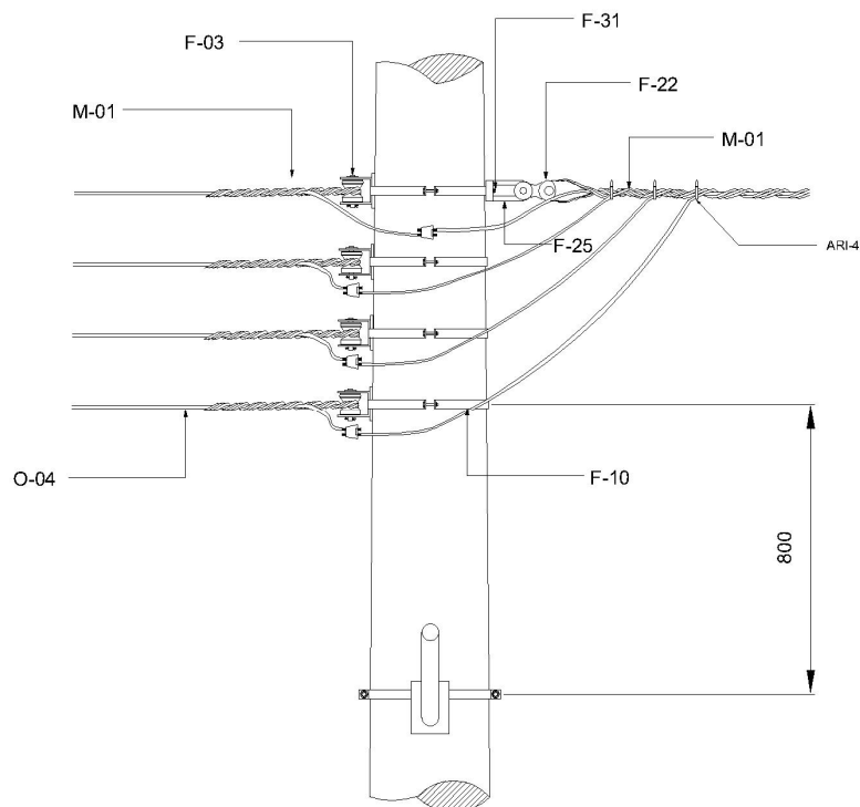
Figura 7 - Estruturas transição rede nua / rede isolada S3 – SI 3
