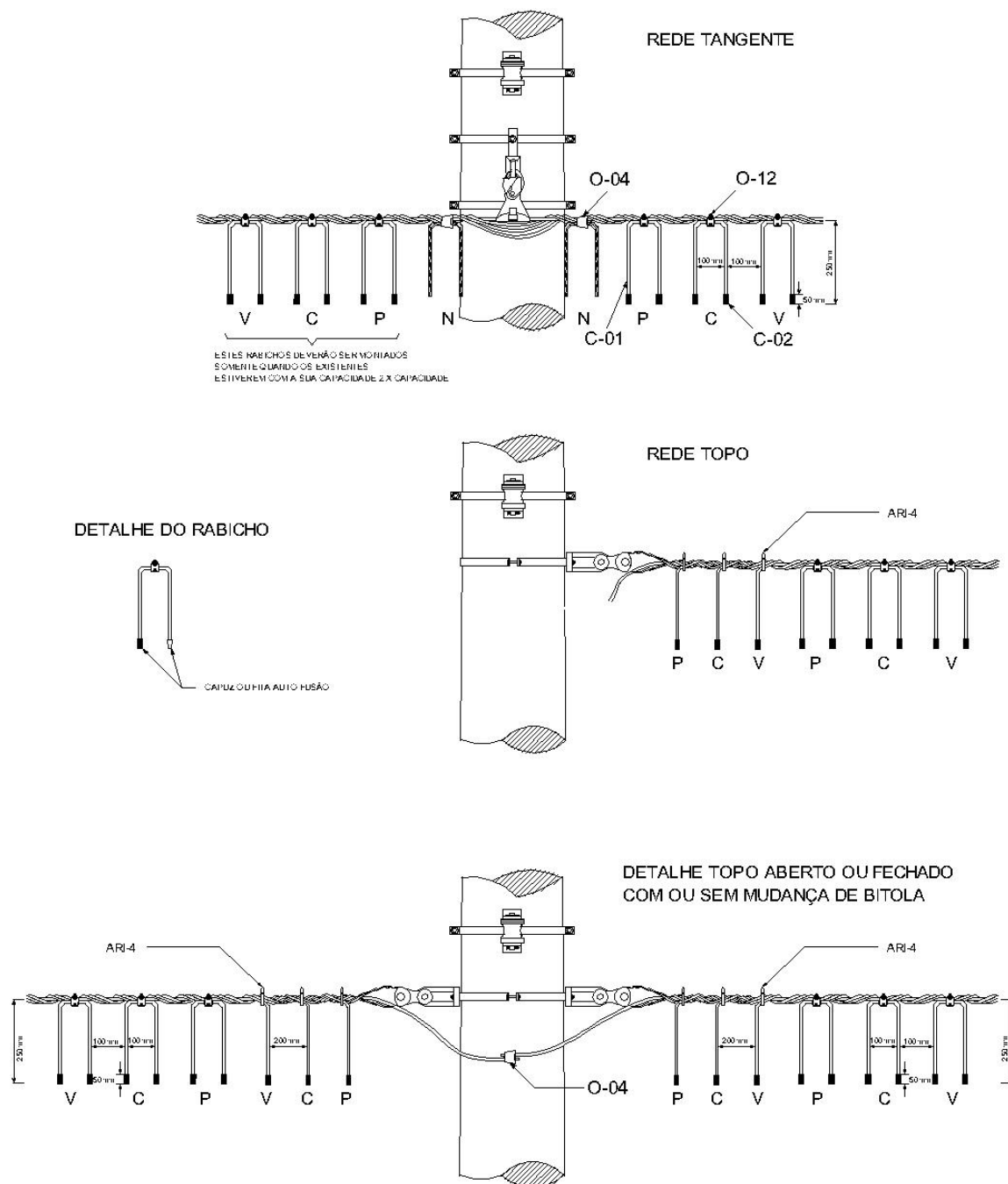
Figura 14 - Identificação das fases – Ligação de clientes
