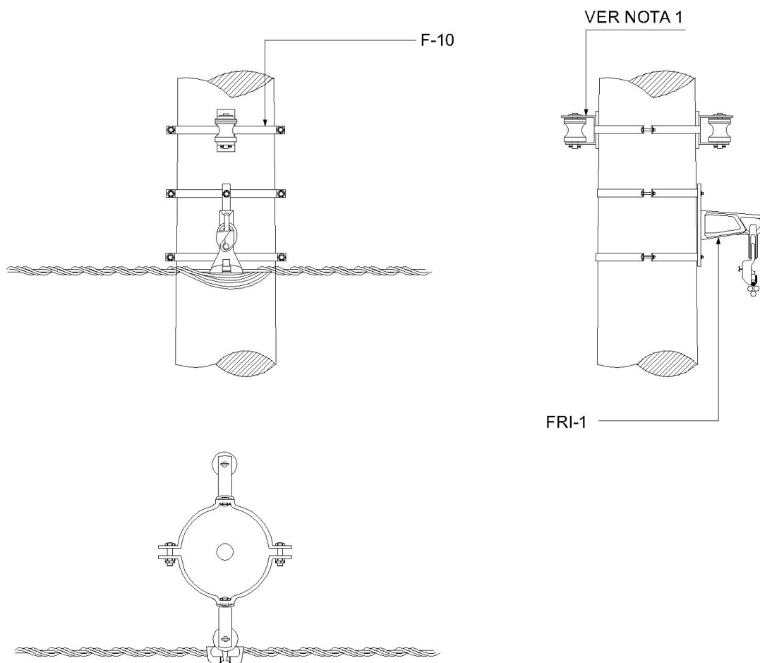
Figura 2 – Estruturas tangentes – SI 1
