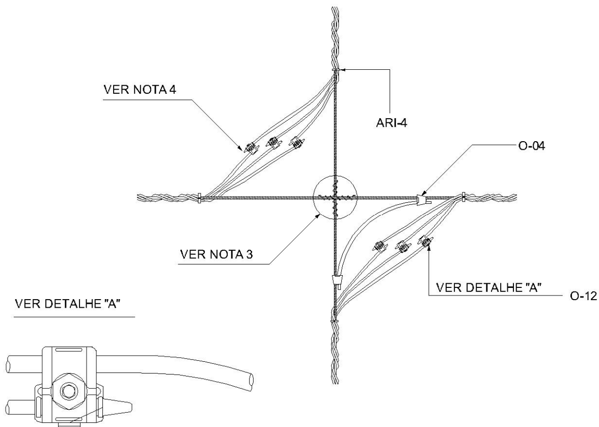
Figura 11 - Estrutura cruzamento sem conexão no vão
