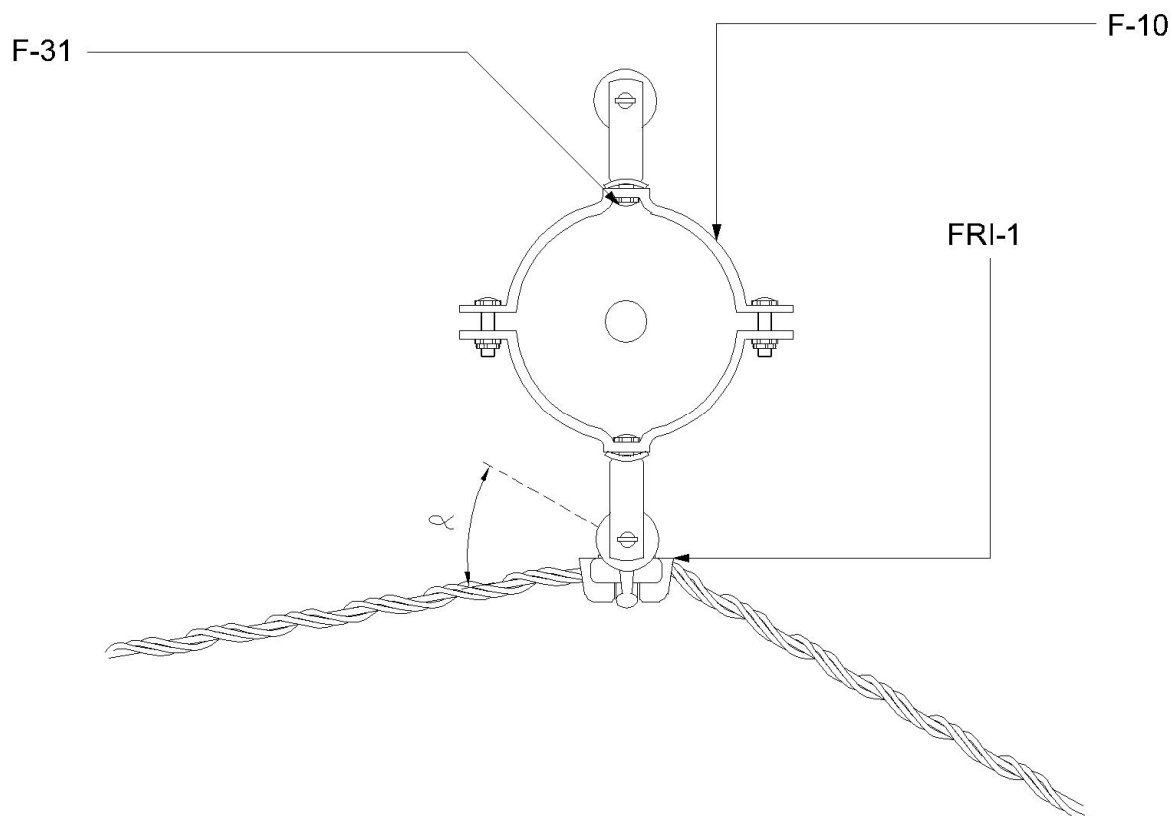
Figura 3 – Estrutura em ângulo – SI 2
