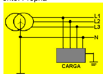
Figura 4 - Esquema TT Fonte: Própria
