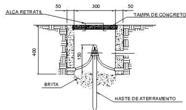
CORTE AA'
